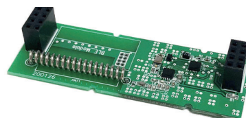
Reception unit - Doorlock
